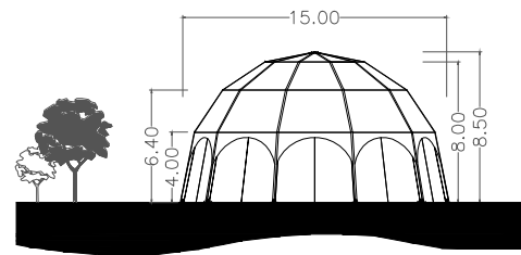
HAUPTANSICHT
