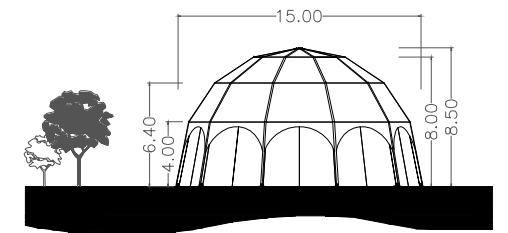
HAUPTANSICHT
