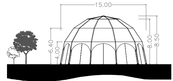
HAUPTANSICHT
