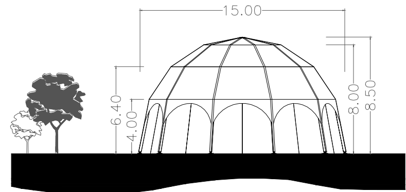
HAUPTANSICHT
