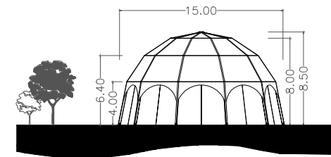
HAUPTANSICHT
