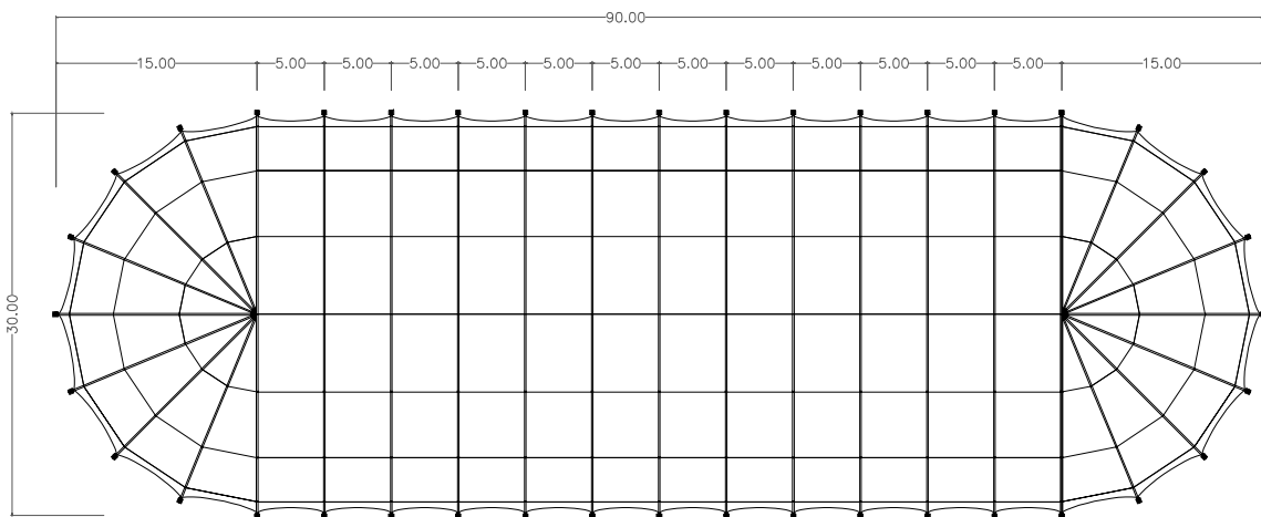
DRAUFSICHT
