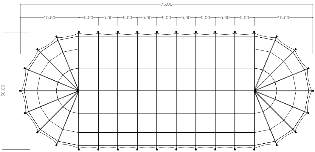
DRAUFSICHT
