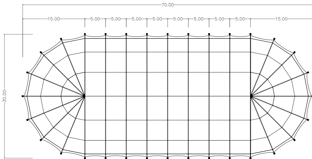
DRAUFSICHT
