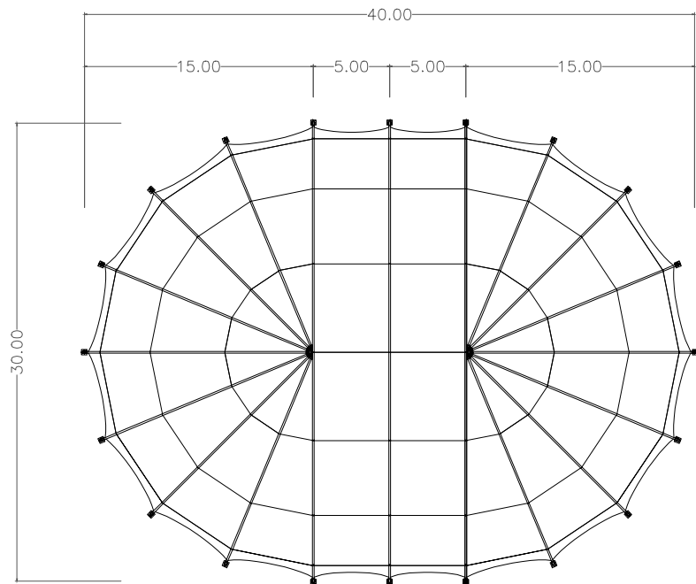
DRAUFSICHT
