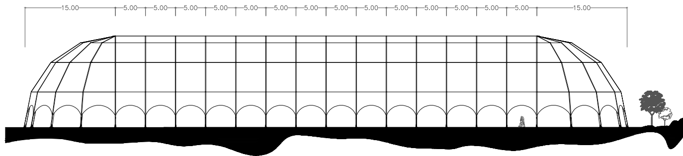
SEITENANSICHT
