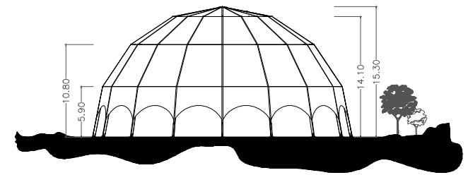
HAUPTANSICHT
