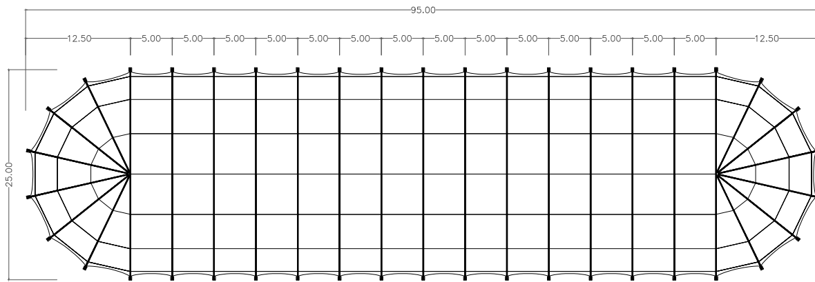
DRAUFSICHT
