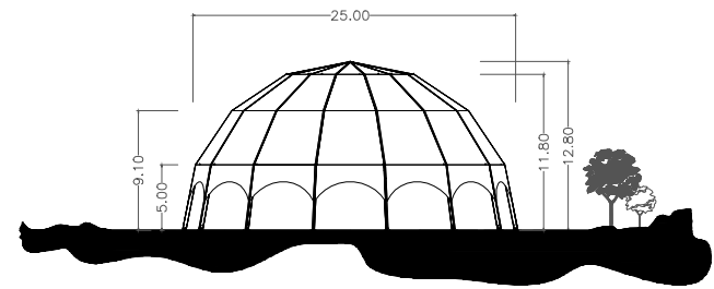
HAUPTANSICHT
