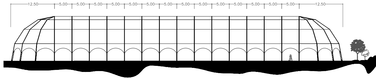
SEITENANSICHT
