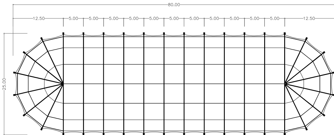
DRAUFSICHT
