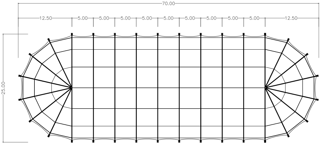
DRAUFSICHT
