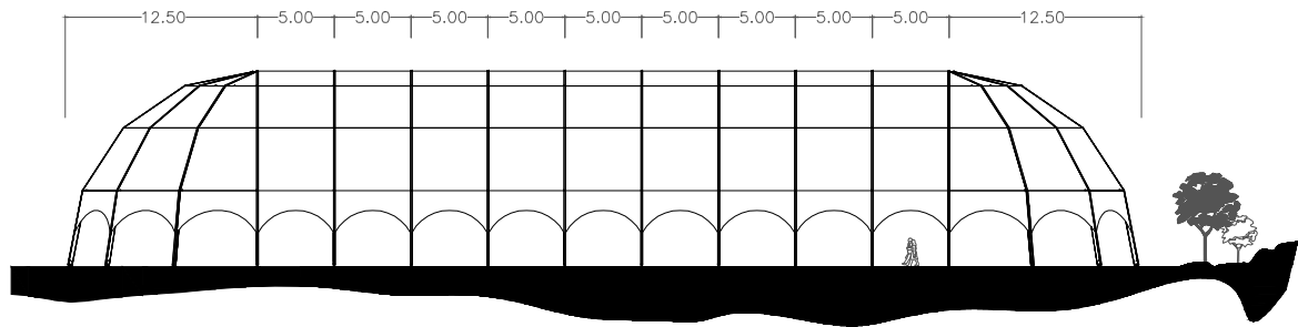
SEITENANSICHT
