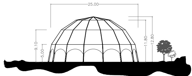
HAUPTANSICHT
