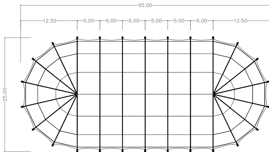
DRAUFSICHT
