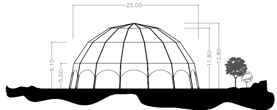
HAUPTANSICHT
