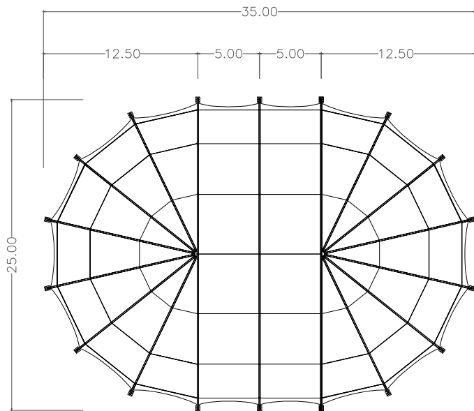
DRAUFSICHT
