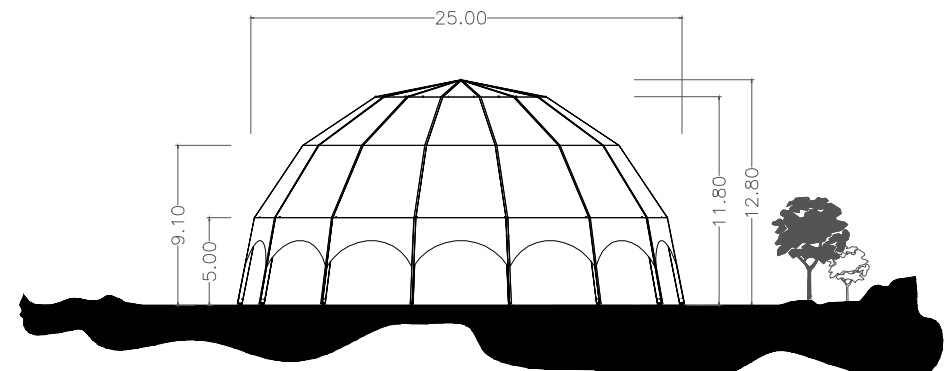
HAUPTANSICHT
