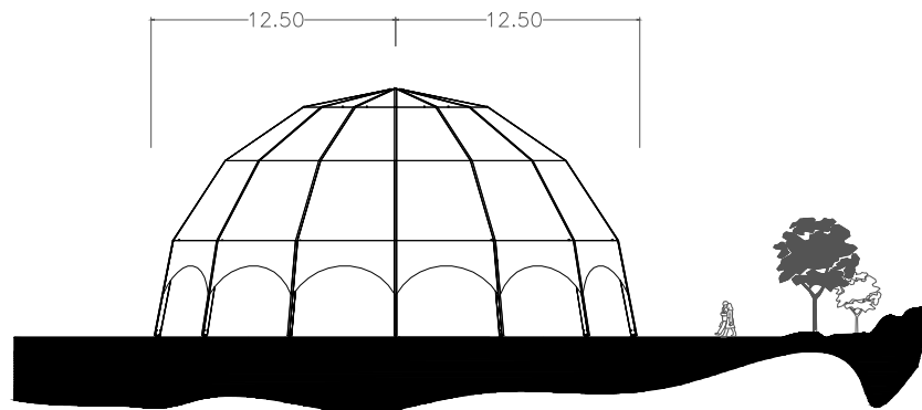
SEITENANSICHT
