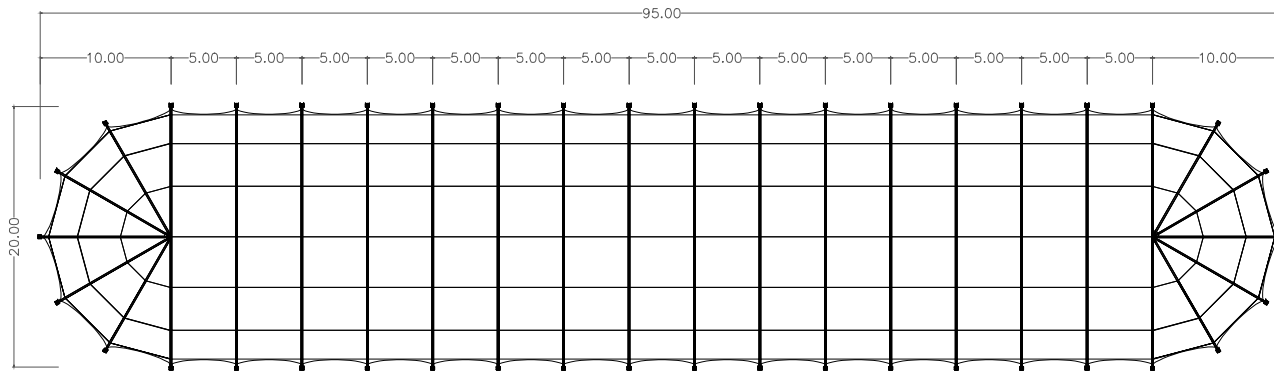
DRAUFSICHT
