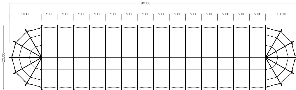
DRAUFSICHT
