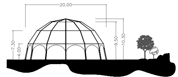
HAUPTANSICHT
