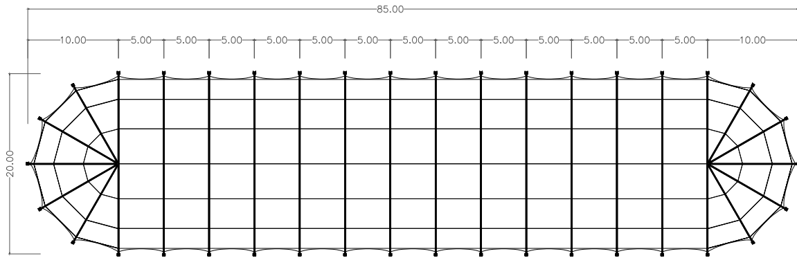
DRAUFSICHT
