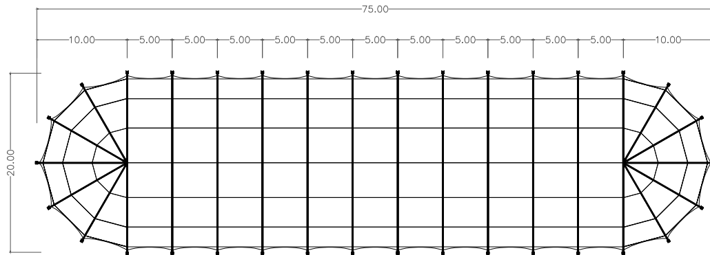
DRAUFSICHT
