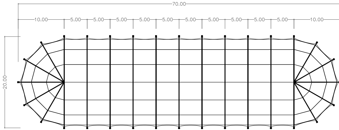
DRAUFSICHT
