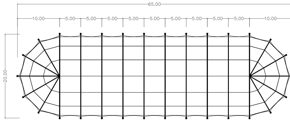
DRAUFSICHT
