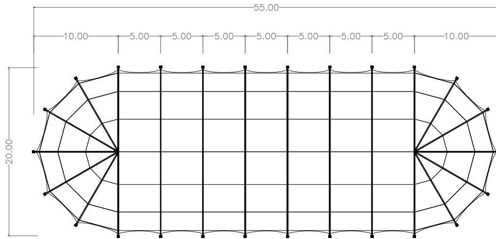
DRAUFSICHT
