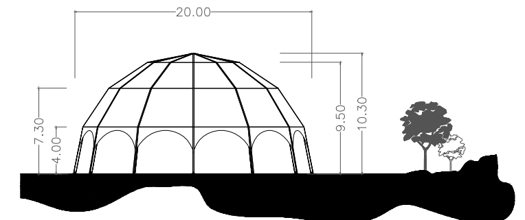
HAUPTANSICHT
