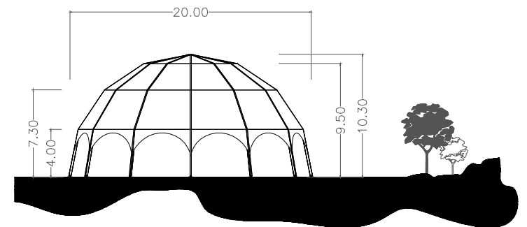
HAUPTANSICHT
