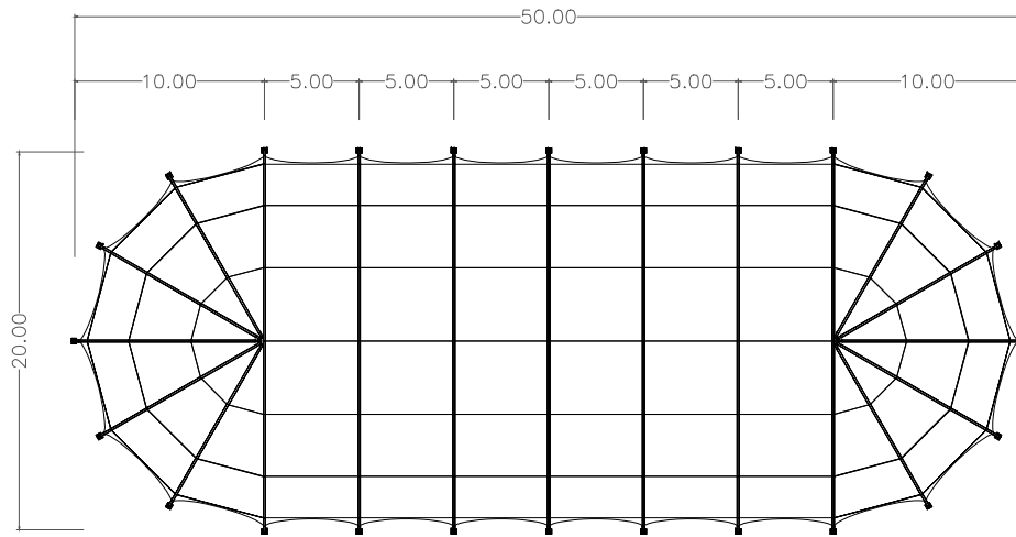
DRAUFSICHT
