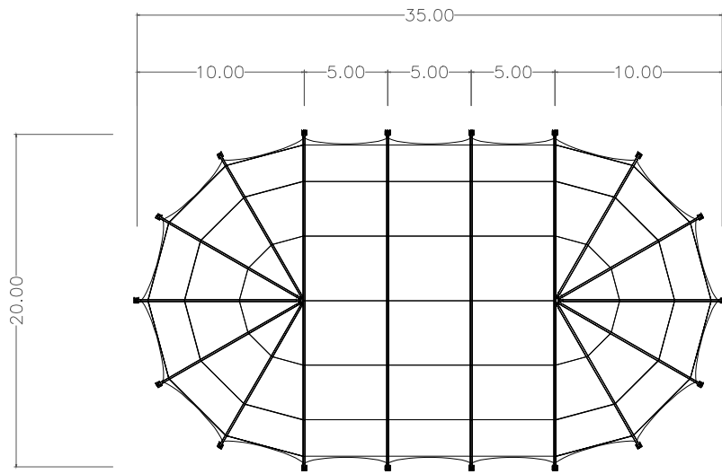
DRAUFSICHT
