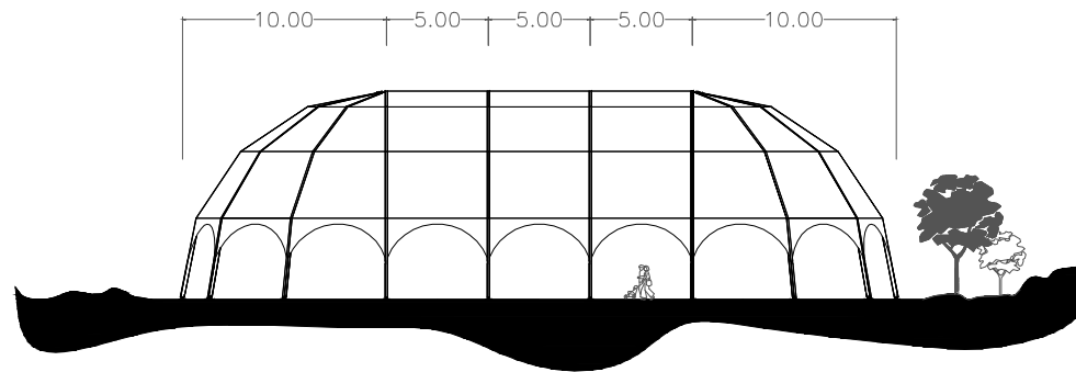
SEITENANSICHT
